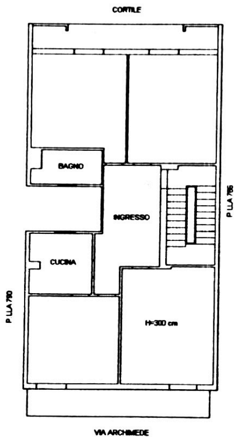
PIANO TERZO
